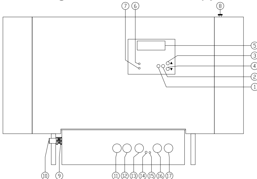
2) Positionszeichnung
